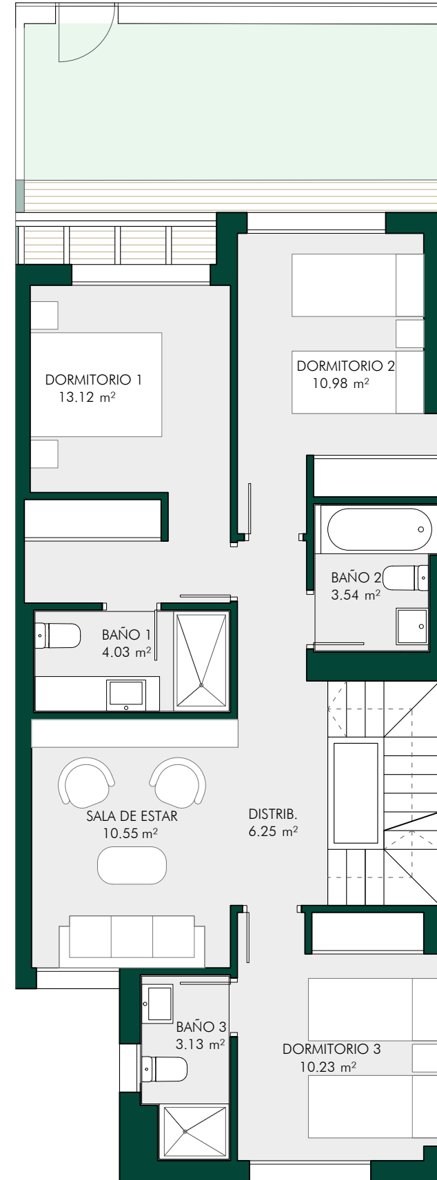
PLANTA PRIMERA
